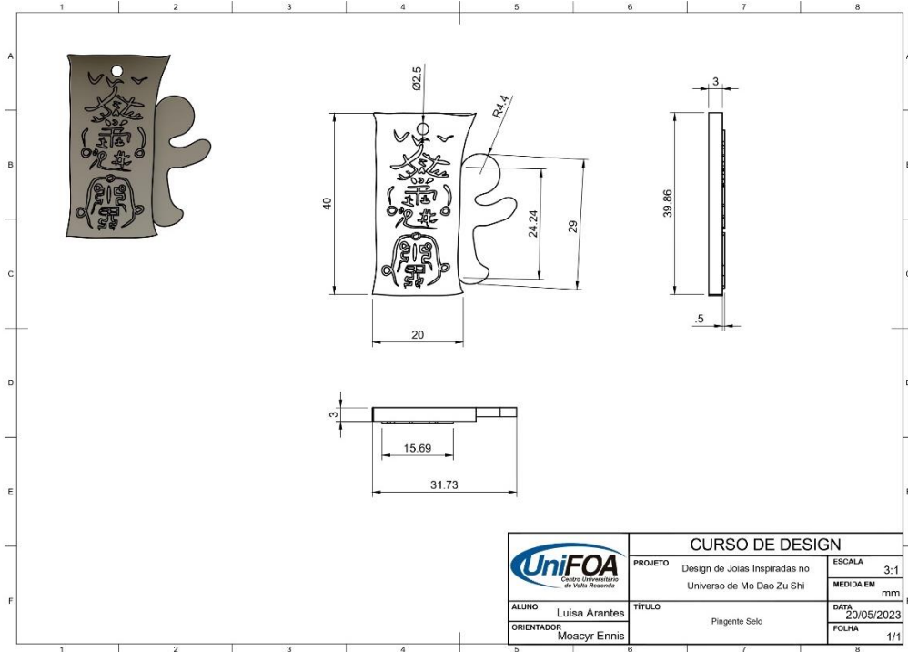
Figura 151 - Desenho Técnico Pingente Selo.
