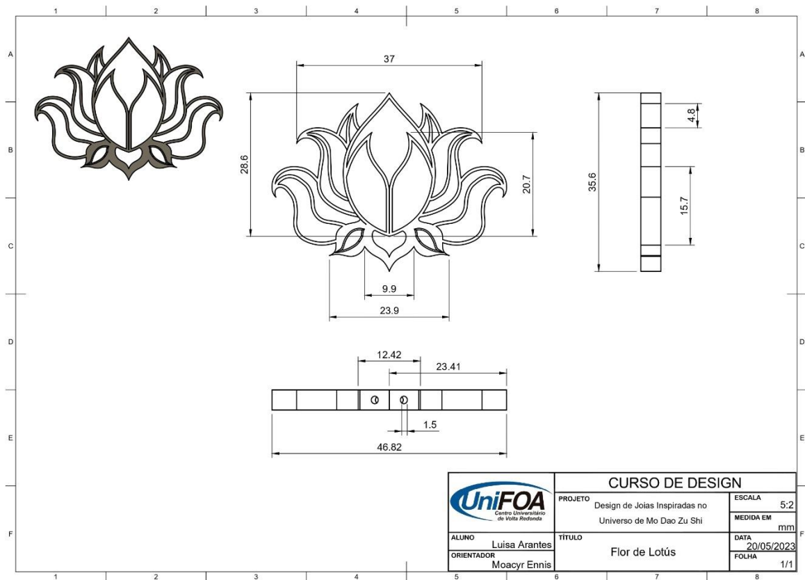
Figura 153 - Desenho Técnico Lotus.
