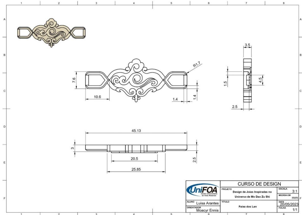
Figura 149 - Desenho Técnico Faixa dos Lan.
