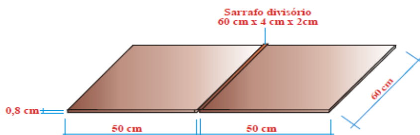
Figura 4 - Dimensões da plataforma de madeira utilizada no teste 3 (CARMINATO, 2010, p. 43)
