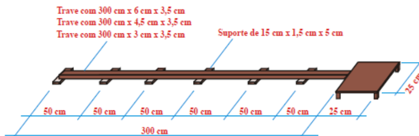
Figura 1 - Dimensões das traves de equilíbrio utilizadas no teste 1 (CARMINATO, 2010, p. 38)
