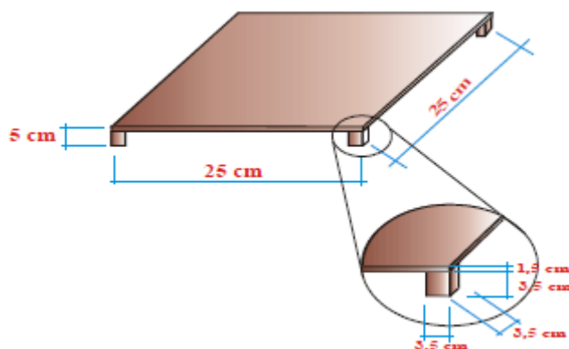
Figura 5 - Dimensões da plataforma de madeira utilizada no teste 4 (CARMINATO, 2010, p. 45)
